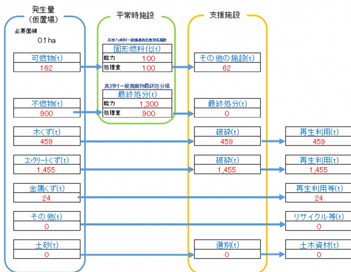
図 2-6-4 留萌沖(走行 N193° E、モデル No.1)地震の災害廃棄物処理フロー
