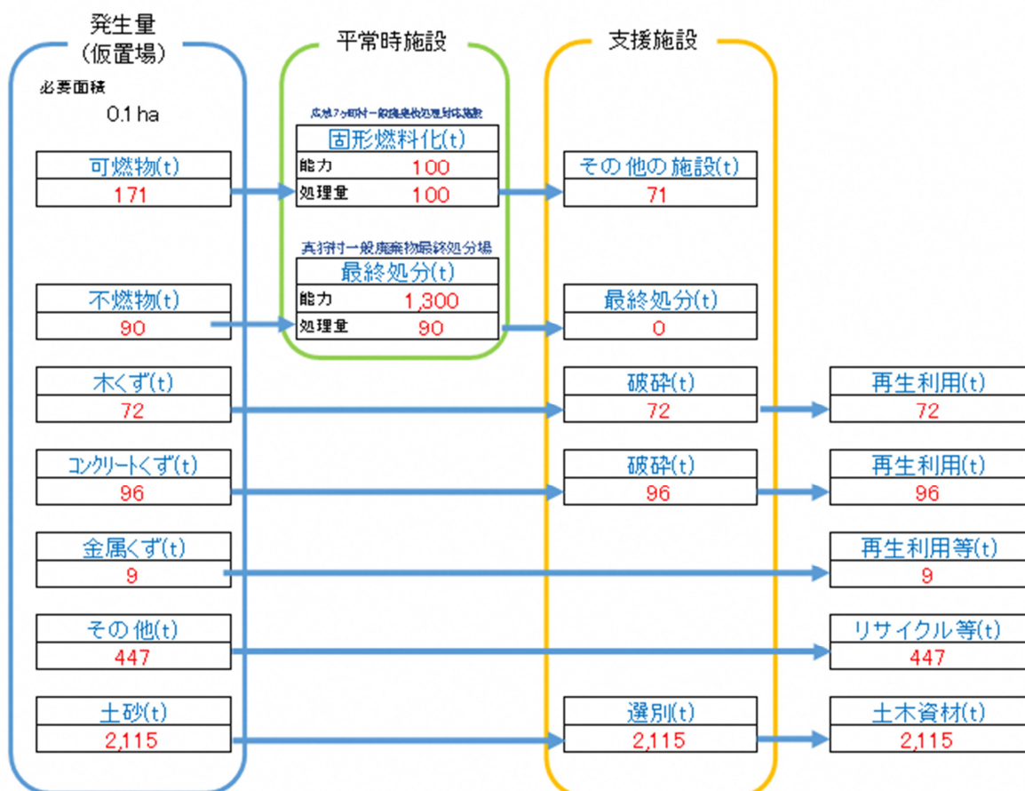
図 2-6-6 真狩村内の土砂災害の災害廃棄物処理フロー
